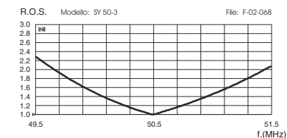
RISPOSTA R.O.S. TIPICA
