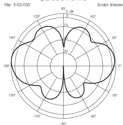
DIAGRAMMA DI RADIAZIONE TIPICO piano E a 145 MHz
